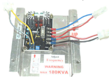
AVR-SE350 Marathon
