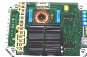
AVR-UVR6 Mecc Alte
