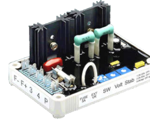
AVR-ND35 Denyo 280
